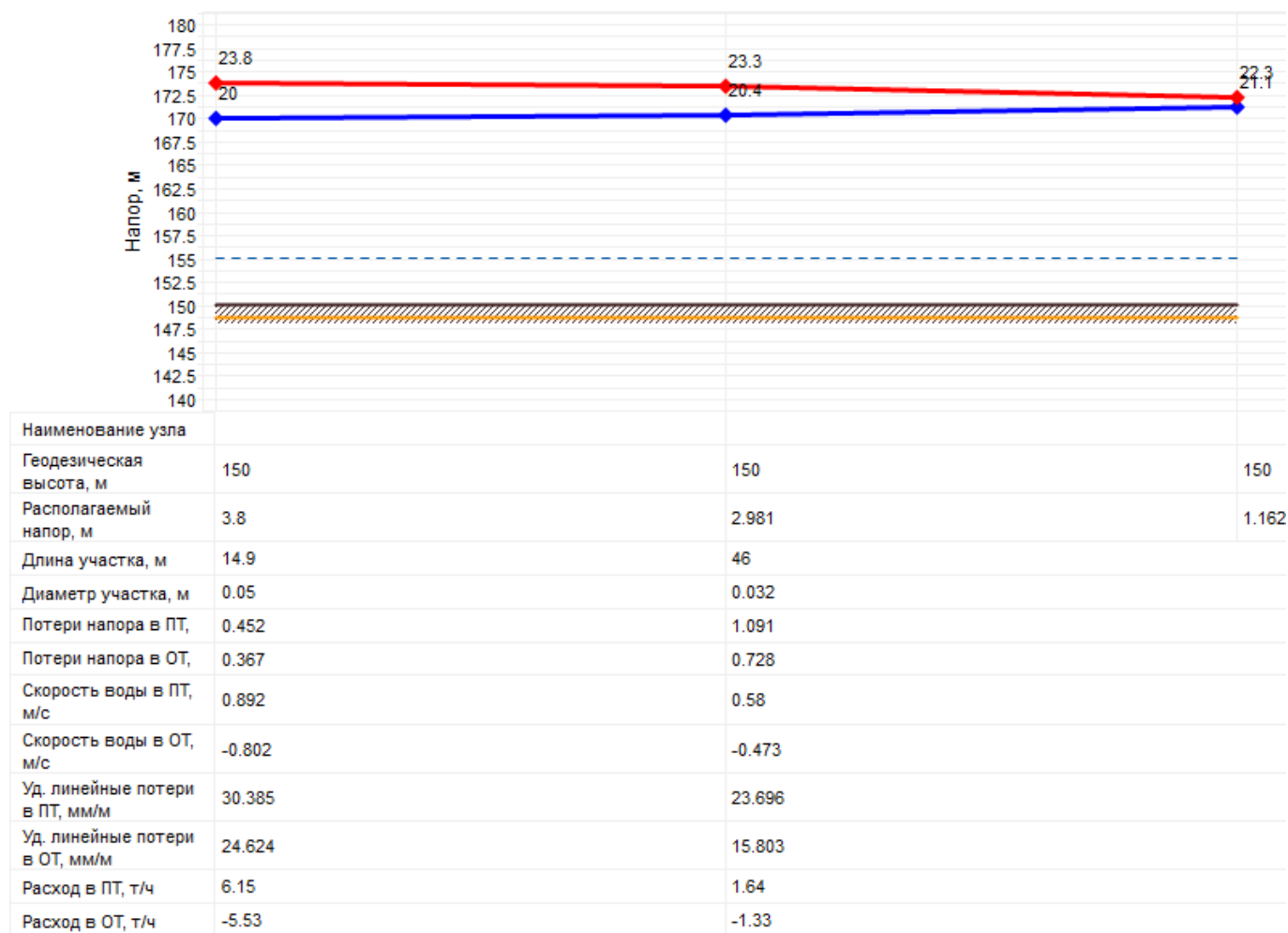
Рисунок 2.11 – Пьезометрический график тепловой сети по магистральному выводу котельной школы
