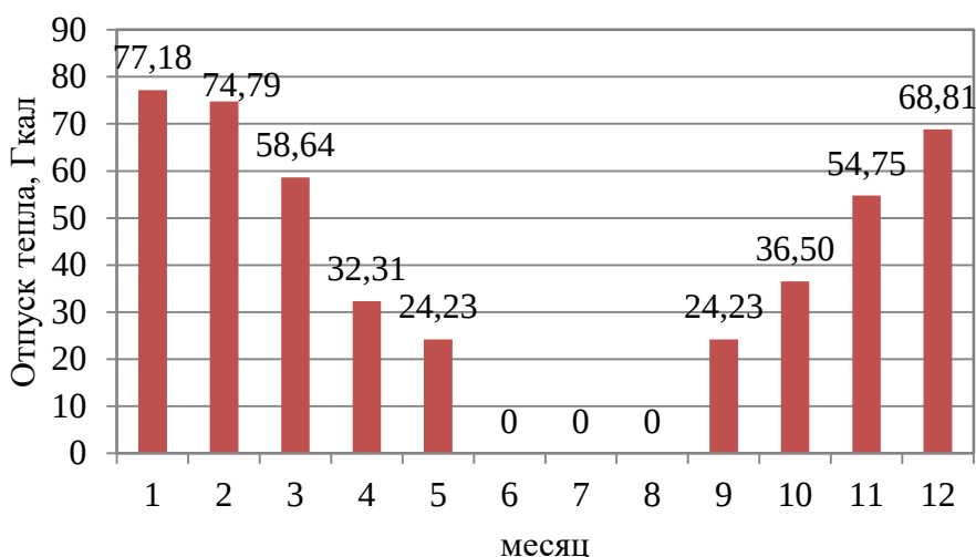
Рисунок 1.15 – Оптимальный температурный график отпуска тепловой энергии для центральной котельной школы с. Введенское
