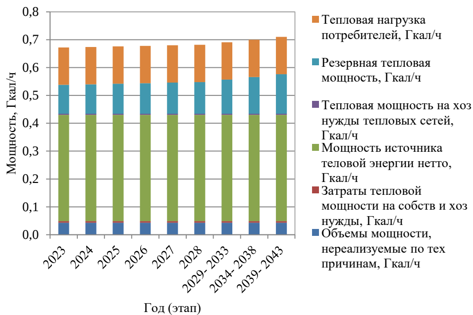
Рисунок 1.13 – Развернутый баланс тепловой мощности и тепловой нагрузки центральной котельной ДРСУ
