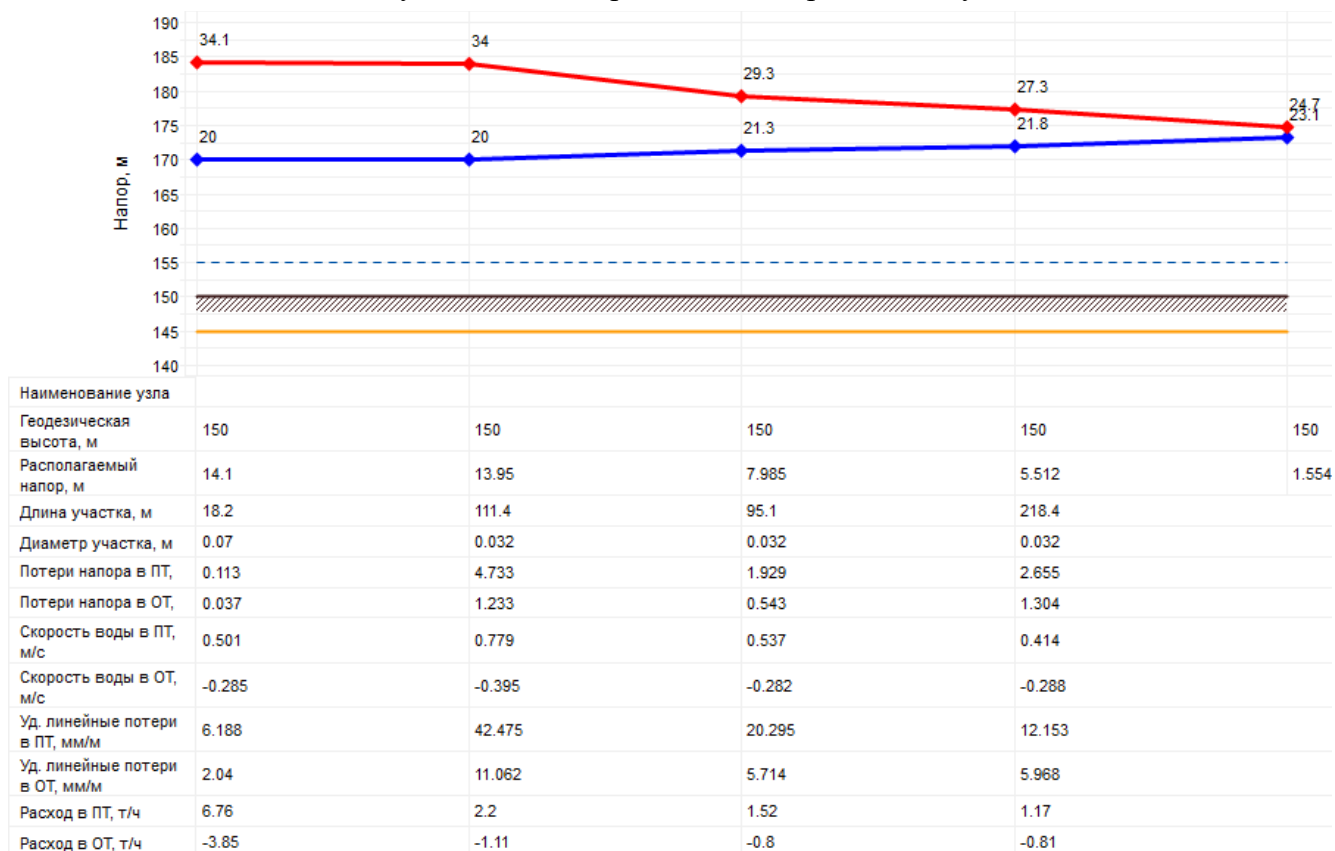
Рисунок 2.24 – Пьезометрический график от источника теплоснабжения (котельной ДРСУ) до самого удаленного потребителя в аварийной ситуации
