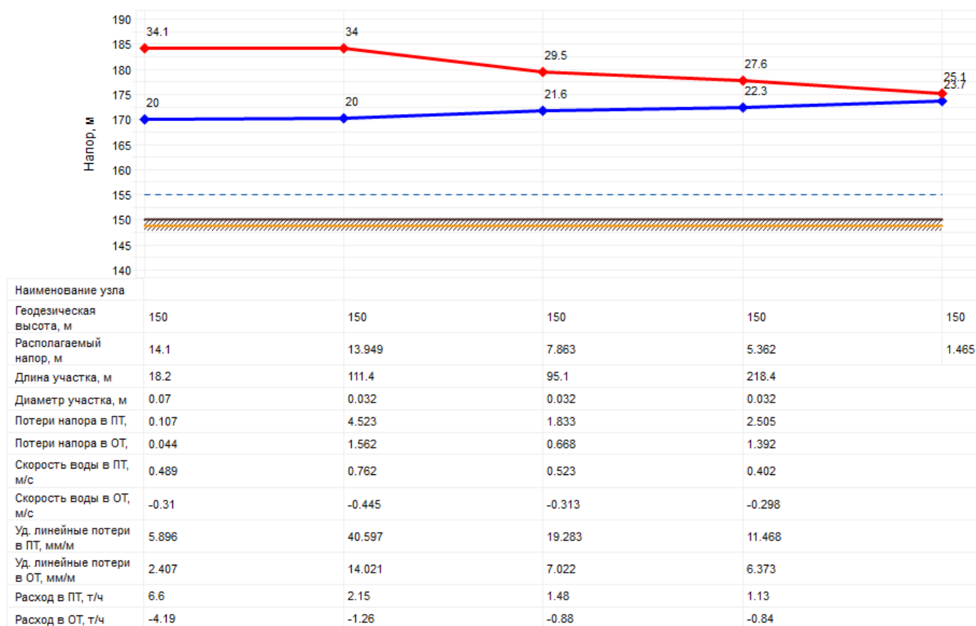
Рисунок 2.6 – Пьезометрический график тепловой сети котельной ДРСУ
