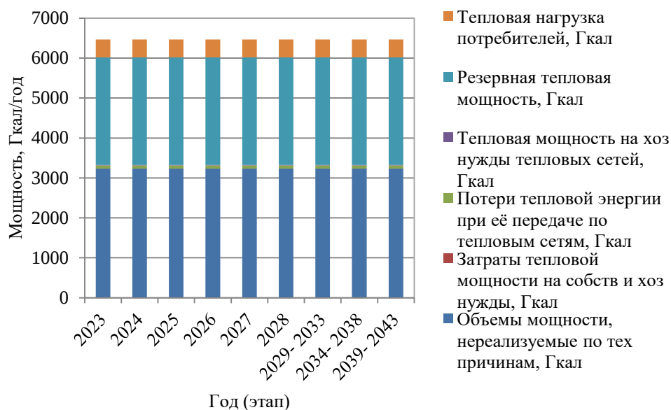
Рисунок 1.10 – Развернутый баланс тепловой энергии и тепловой нагрузки центральной котельной школы
