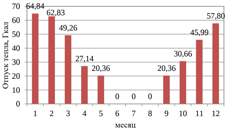
Рисунок 1.16 – Оптимальный температурный график отпуска тепловой энергии для котельной больницы с. Введенское
