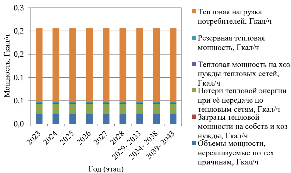
Рисунок 1.11 – Развернутый баланс тепловой мощности и тепловой нагрузки центральной котельной больницы
