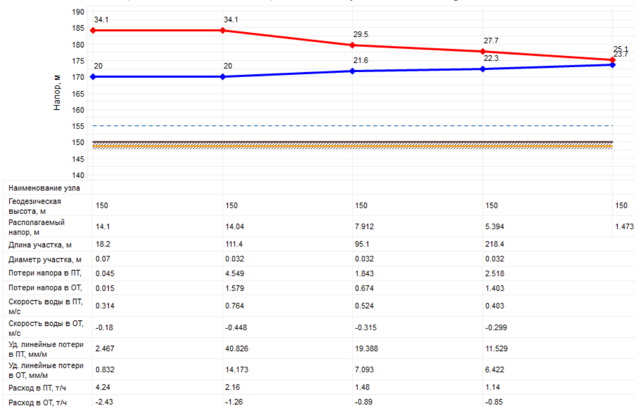
Рисунок 2.21 – Пьезометрический график от источника теплоснабжения (котельной ДРСУ) до самого удаленного потребителя
