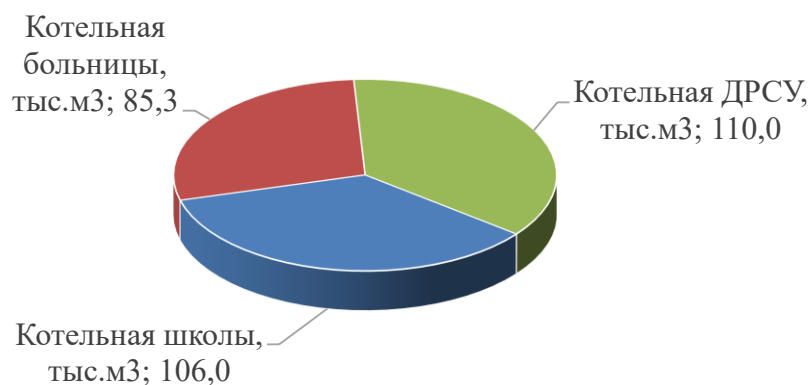
Рисунок 2.14 – Доля топлива используемого для производства тепловой энергии по системам теплоснабжения
