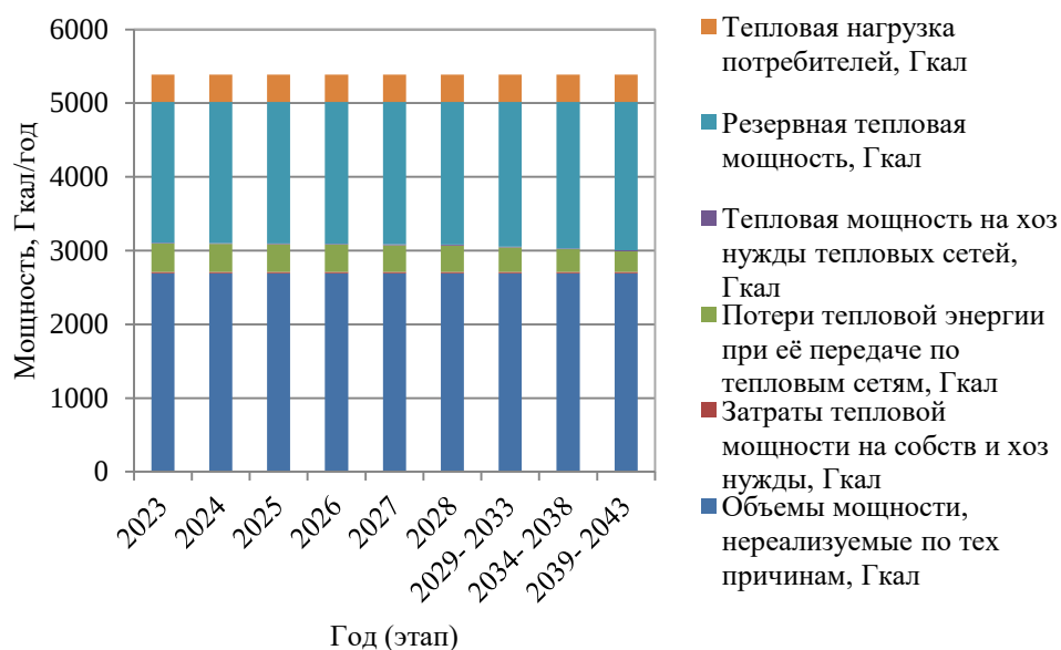
Рисунок 1.14 – Развернутый баланс тепловой энергии и тепловой нагрузки центральной котельной ДРСУ
