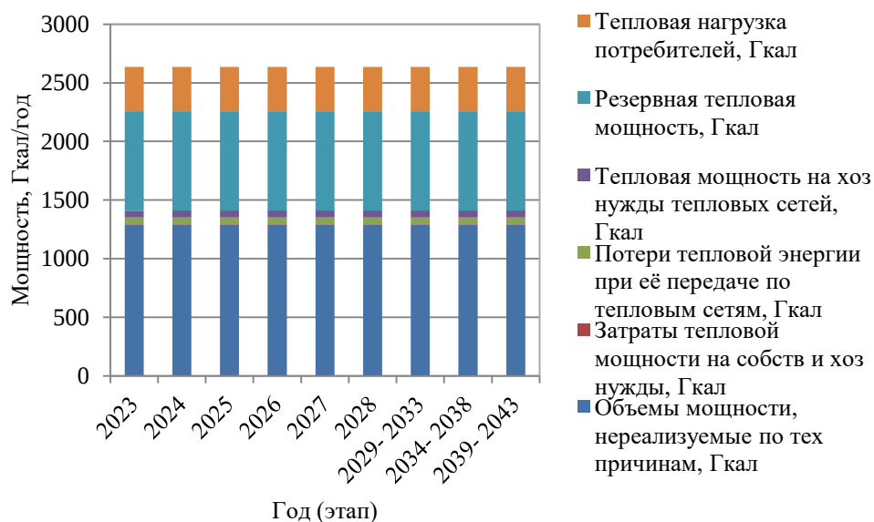
Рисунок 1.12 – Развернутый баланс тепловой энергии и тепловой нагрузки центральной котельной больницы
