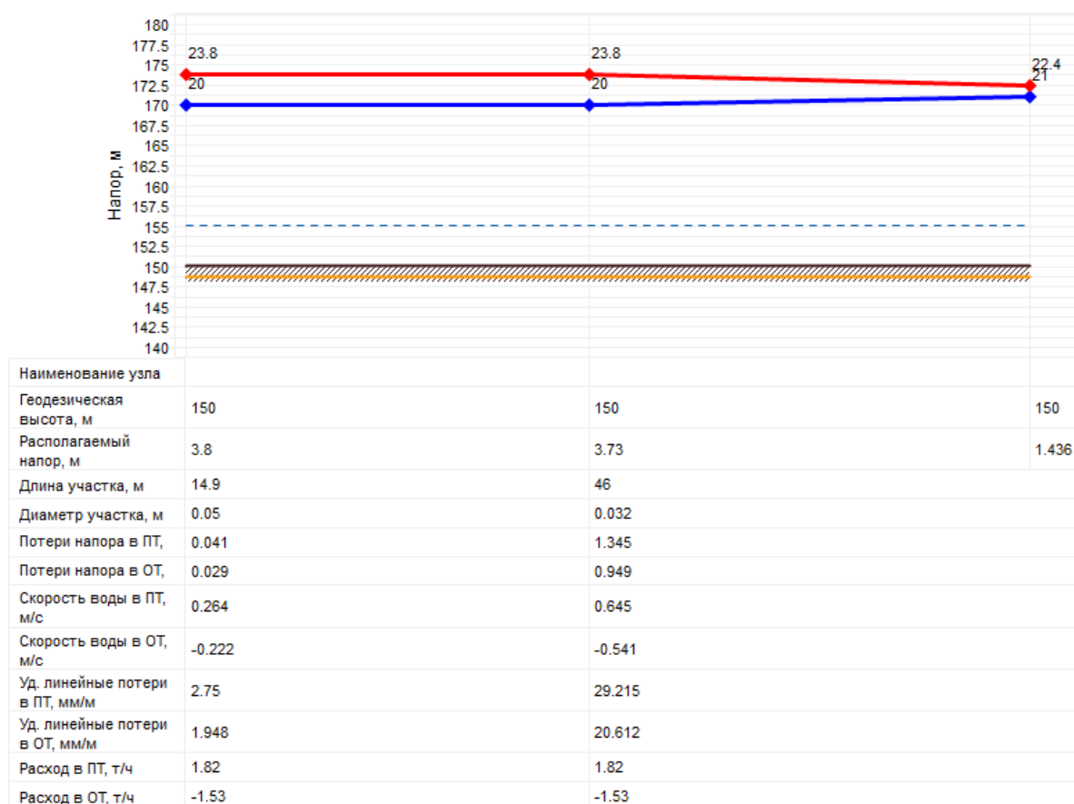
Рисунок 2.19 – Пьезометрический график от источника теплоснабжения (котельной школы) до самого удаленного потребителя
