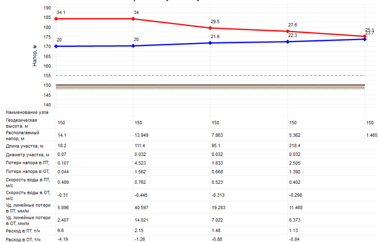
Рисунок 2.13 – Пьезометрический график тепловой сети по магистральному выводу котельной ДРСУ
