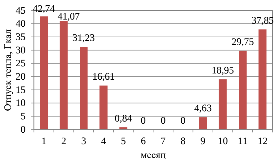
Рисунок 1.17 – Оптимальный температурный график отпуска тепловой энергии для железнодорожной котельной ДРСУ с. Введенское
