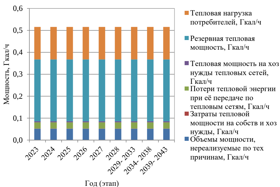
Рисунок 1.9 – Развернутый баланс тепловой мощности и тепловой нагрузки центральной котельной школы
