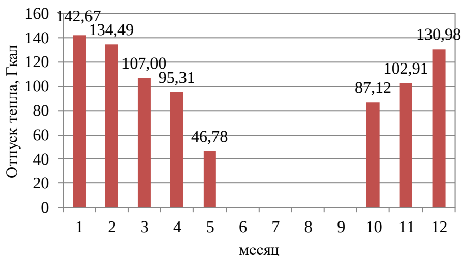
Рисунок 1.6 – Оптимальный температурный график отпуска тепловой энергии центральной котельной с. Колташево
