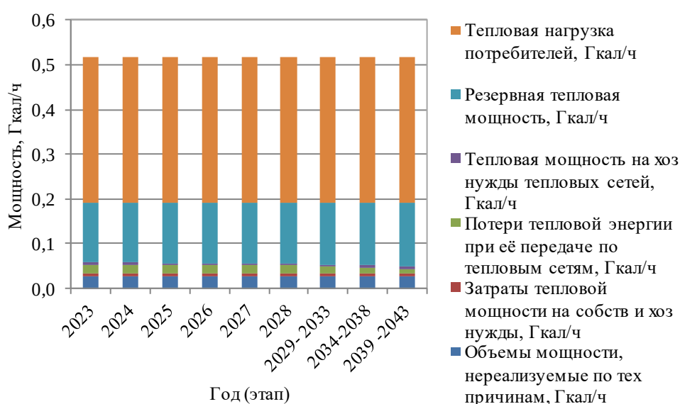
Рисунок 1.4 – Развернутый баланс тепловой мощности и тепловой нагрузки центральной котельной с. Колташево
