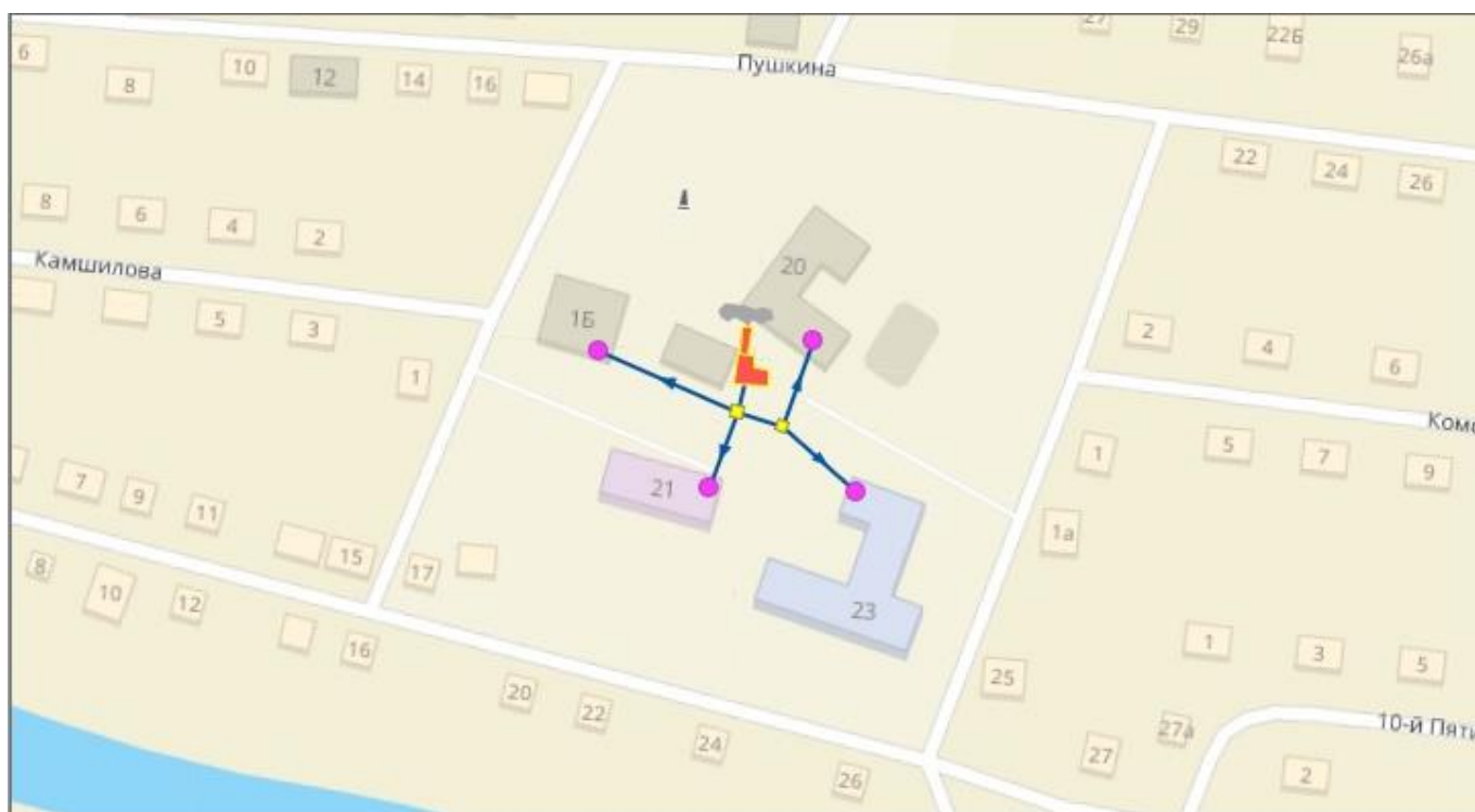
Рисунок 2.4 – Модель системы теплоснабжения котельной с. Колташево
