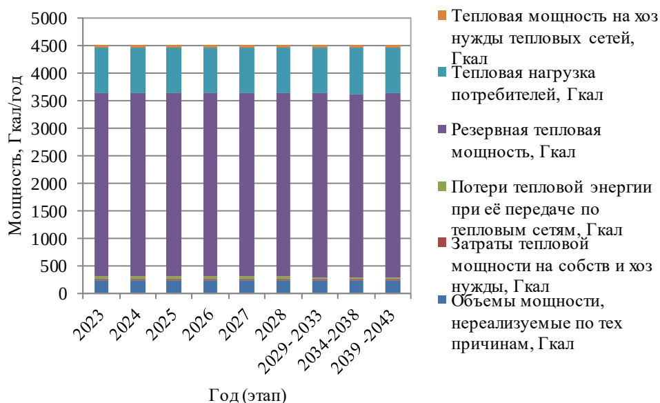
Рисунок 1.5 – Развернутый баланс тепловой энергии и тепловой нагрузки центральной котельной с. Колташево
