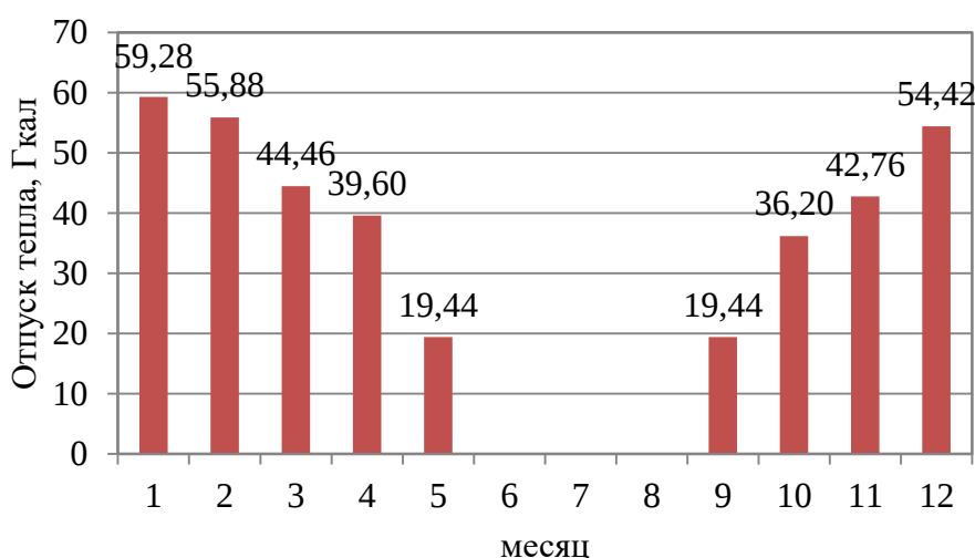
Рисунок 1.6 – Оптимальный температурный график отпуска тепловой энергии для котельной с. Митино
