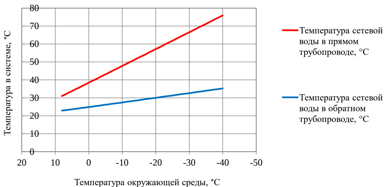
Рисунок 2.2 – График изменения температур теплоносителя
