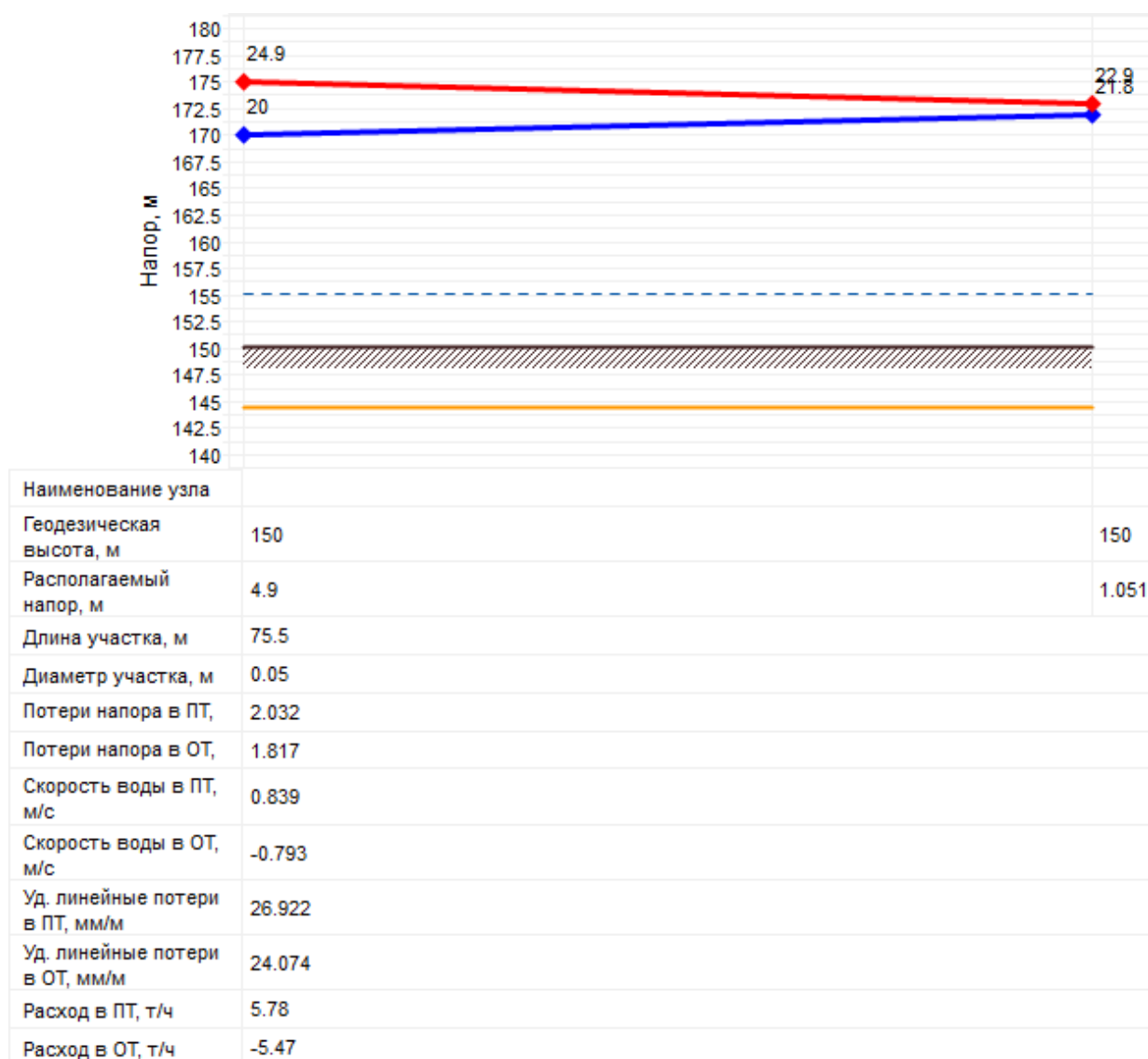
Рисунок 2.8 – Пьезометрический график от источника теплоснабжения (котельной с. Митино) до самого удаленного потребителя в аварийной ситуации
