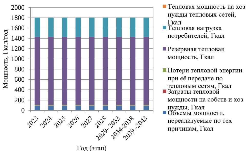
Рисунок 1.5 – Развернутый баланс тепловой энергии и тепловой нагрузки центральной котельной с. Митино
