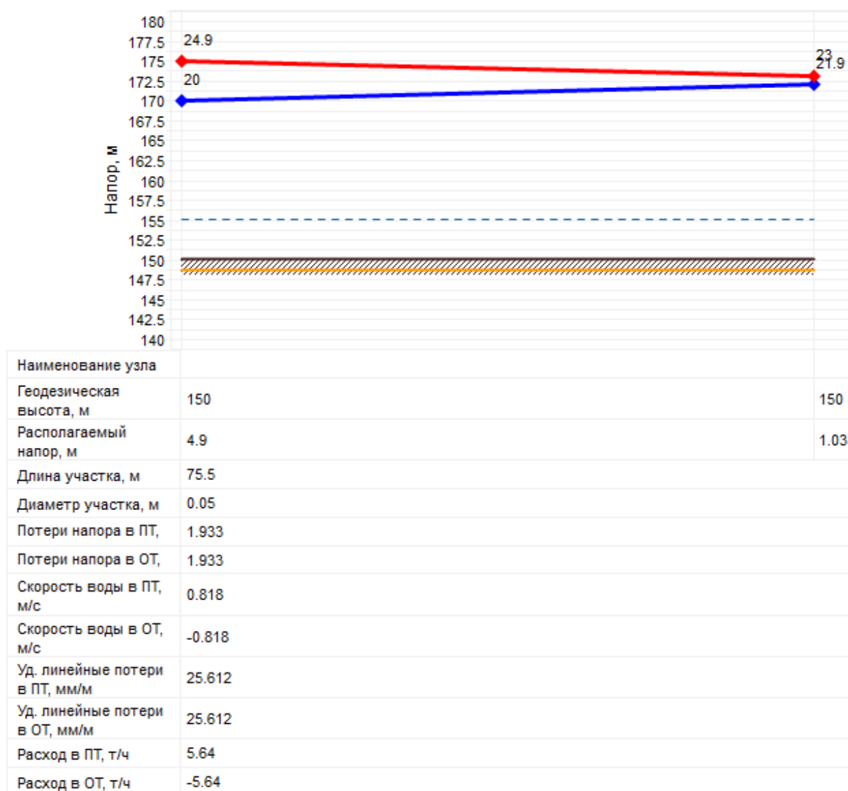
Рисунок 2.3 – Пьезометрический график тепловой сети котельной с. Митино
