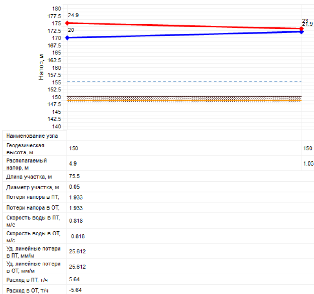
Рисунок 2.5 – Пьезометрический график тепловой сети котельной с. Митино
