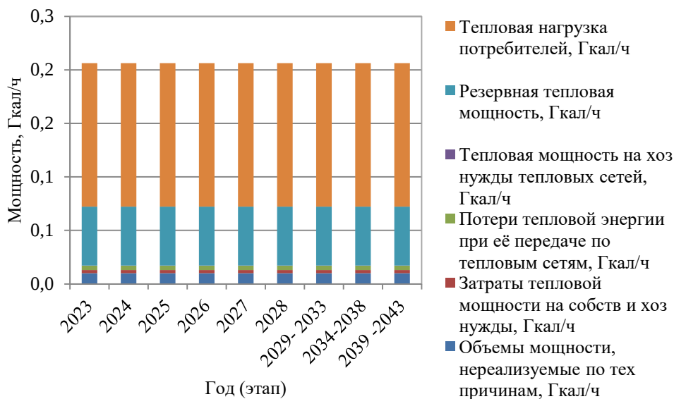
Рисунок 1.4 – Развернутый баланс тепловой мощности и тепловой нагрузки центральной котельной с. Митино
