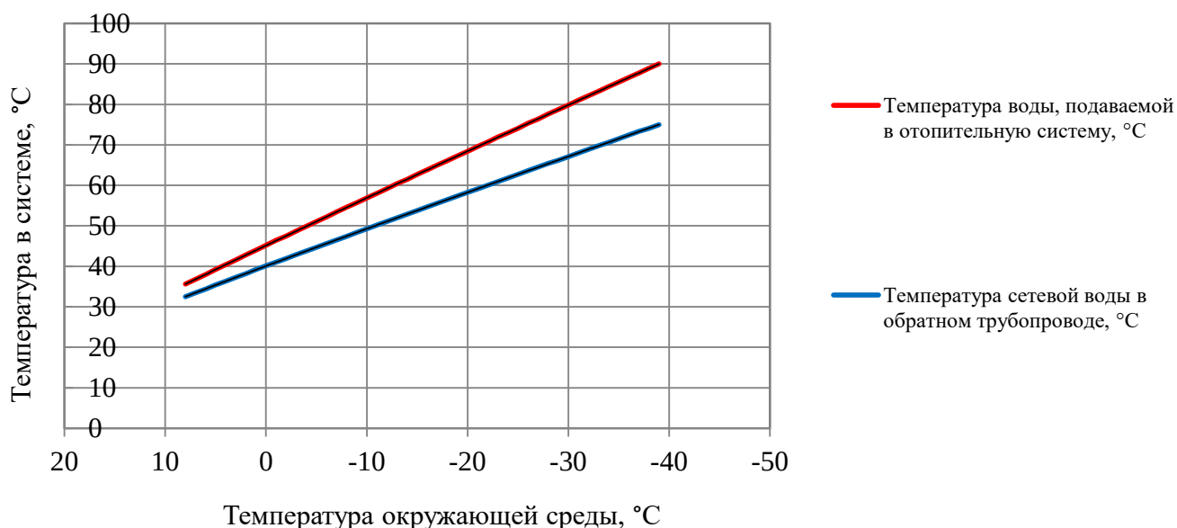
Рисунок 2.2 – График изменения температур теплоносителя
