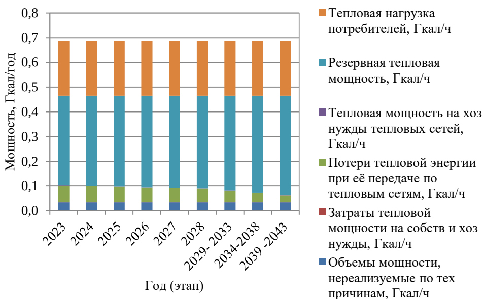
Рисунок 1.4 – Развернутый баланс тепловой мощности и тепловой нагрузки центральной котельной с. Садовое
