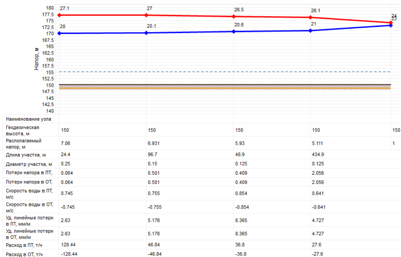
Рисунок 2.3 – Пьезометрический график тепловой сети центральной котельной с. Садовое
