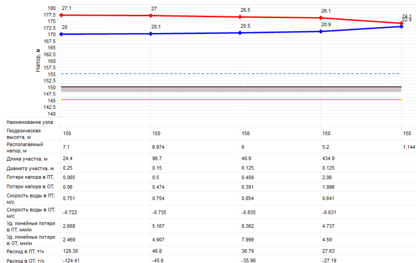
Рисунок 2.9 – Пьезометрический график от источника теплоснабжения (котельной с. Садовое) до самого удаленного потребителя в аварийной ситуации
