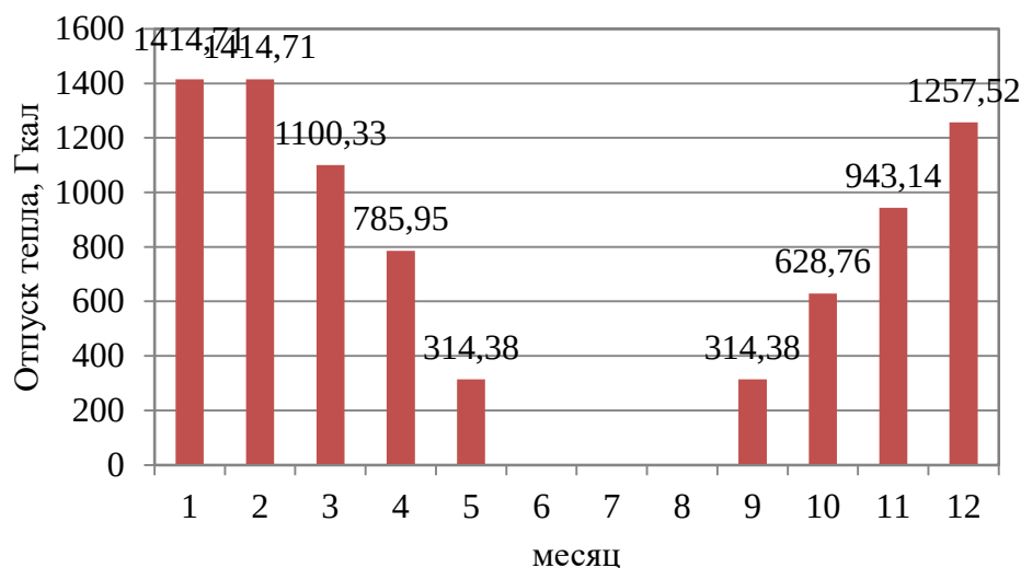
Рисунок 1.6 – Оптимальный температурный график отпуска тепловой энергии центральной котельной с. Садовое до 2026 г.
