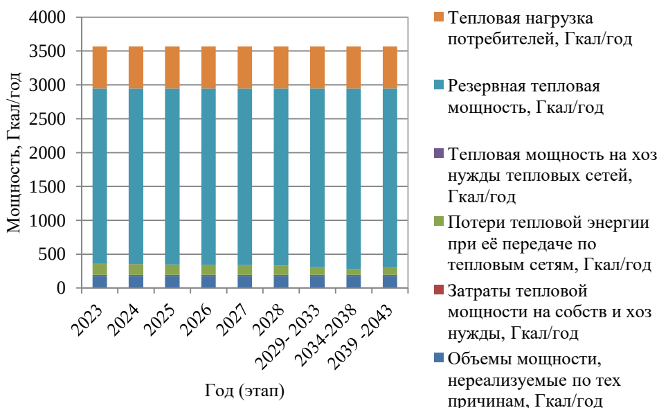
Рисунок 1.5 – Развернутый баланс тепловой энергии и тепловой нагрузки центральной котельной с. Садовое
