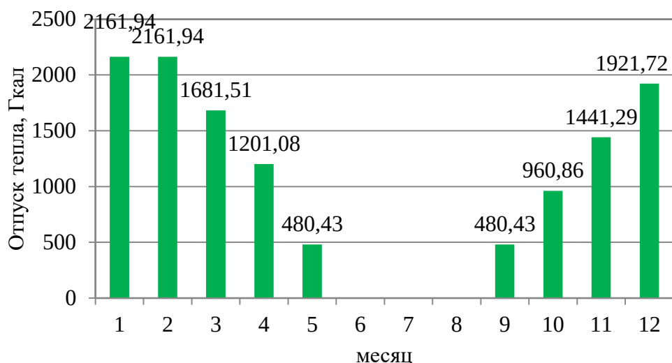
Рисунок 1.7 – Оптимальный температурный график отпуски тепловой энергии центральной котельной с. Садовое к 2043 г.
