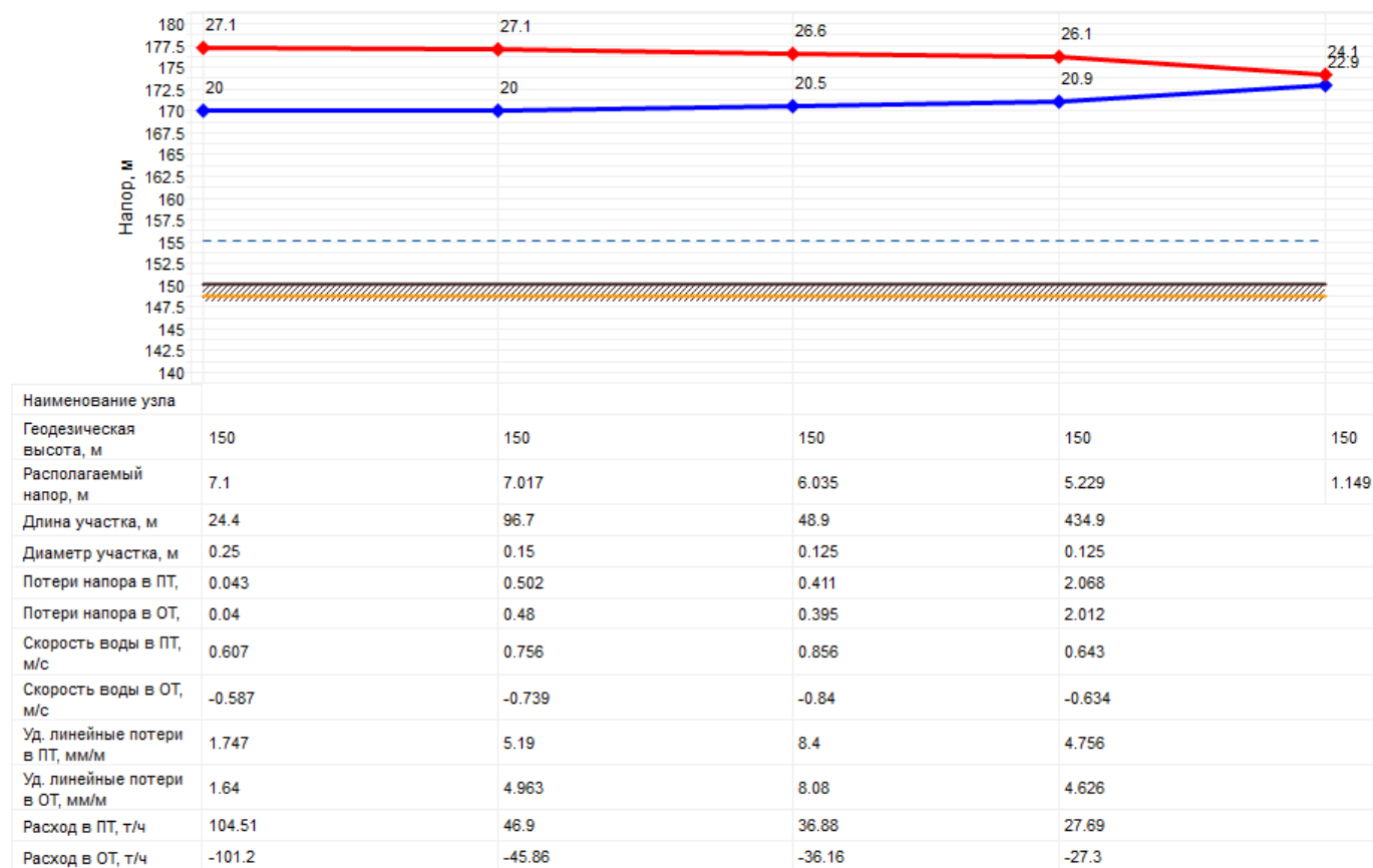
Рисунок 2.8 – Пьезометрический график от источника теплоснабжения (котельной с. Садовое) до самого удаленного потребителя
