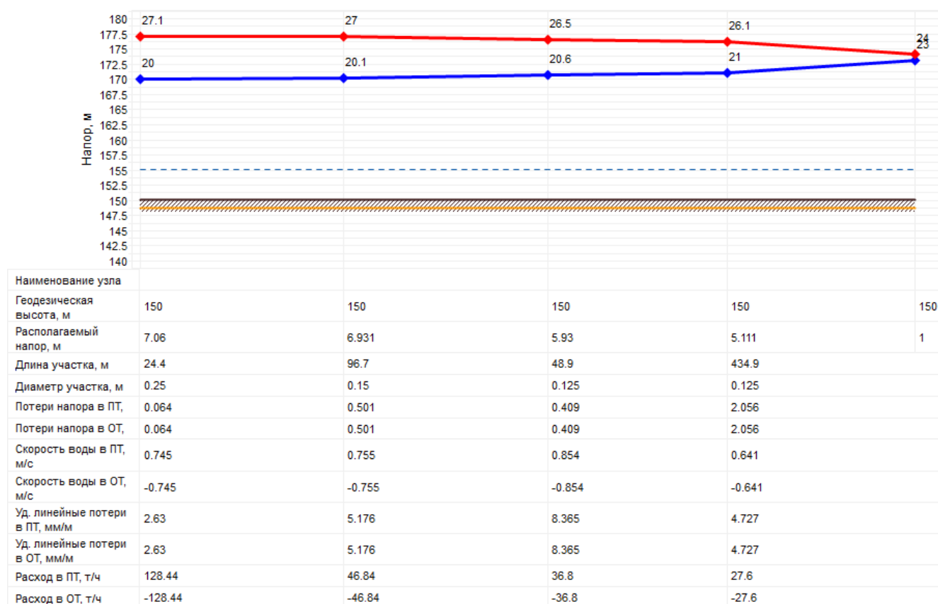
Рисунок 2.5 – Пьезометрический график тепловой сети по магистральному выводу центральной котельной с. Садовое
