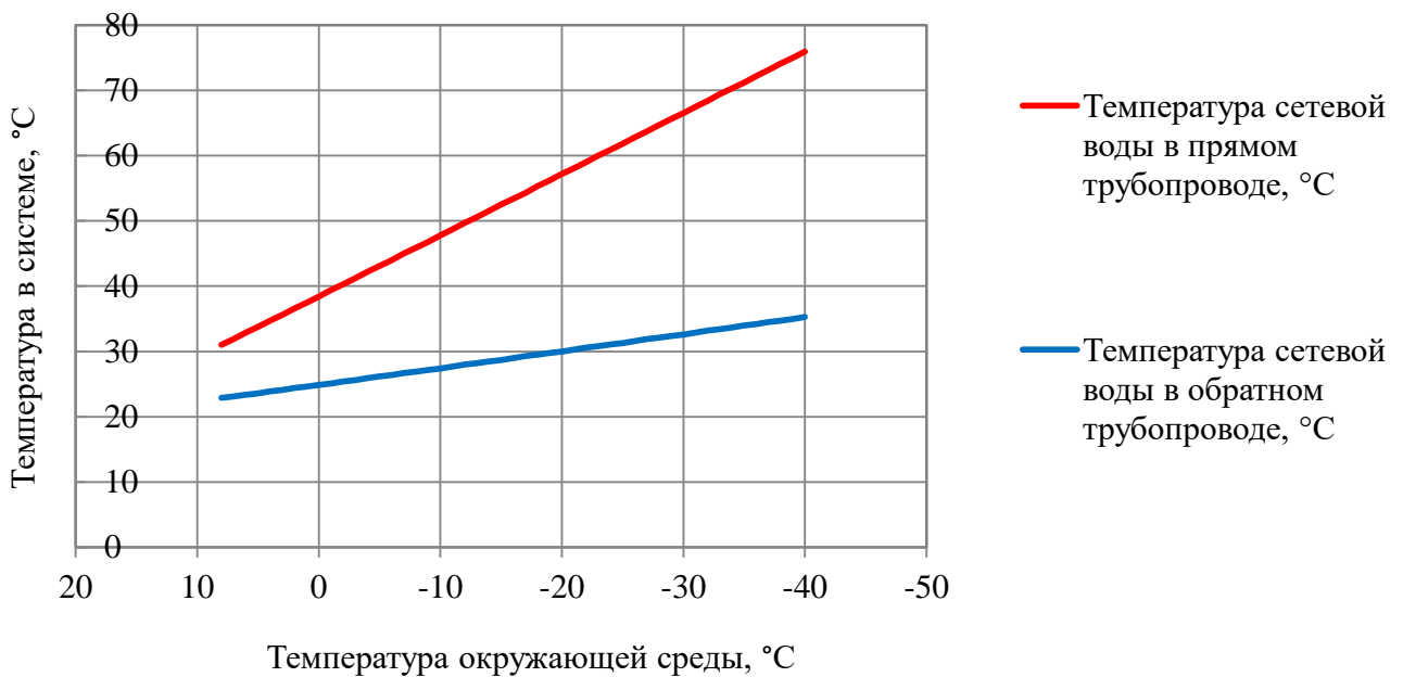
Рисунок 2.2 – График изменения температур теплоносителя
