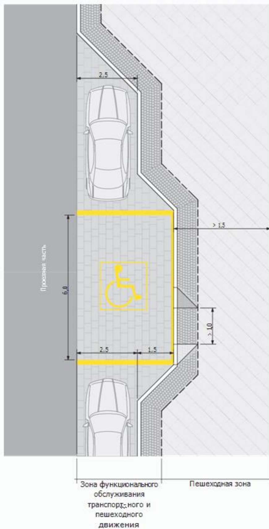
Схема 4
