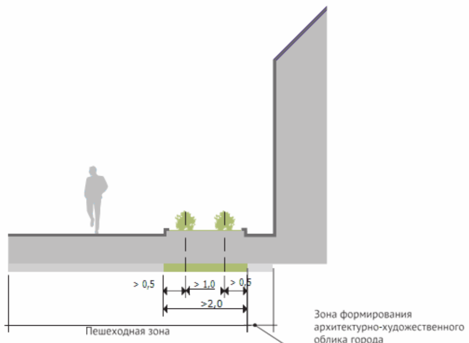
Схема 2
