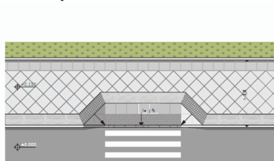
Схема 3–1. Пример организации предупреждающих покрытий при помощи изменения цвета, фактуры и типа укладки
