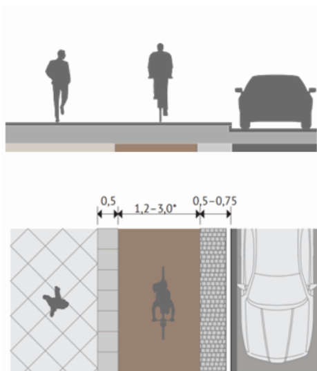
Размещение велодорожки в пешеходной зоне
