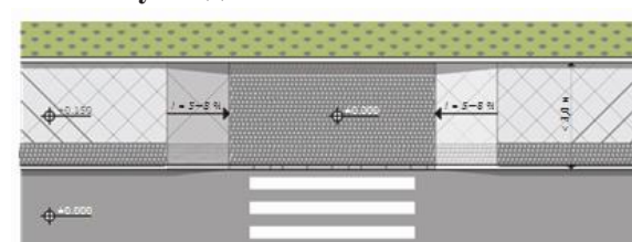
Схема 4–2. Пример организации предупреждающих покрытий при помощи изменения цвета, фактуры и типа укладки
