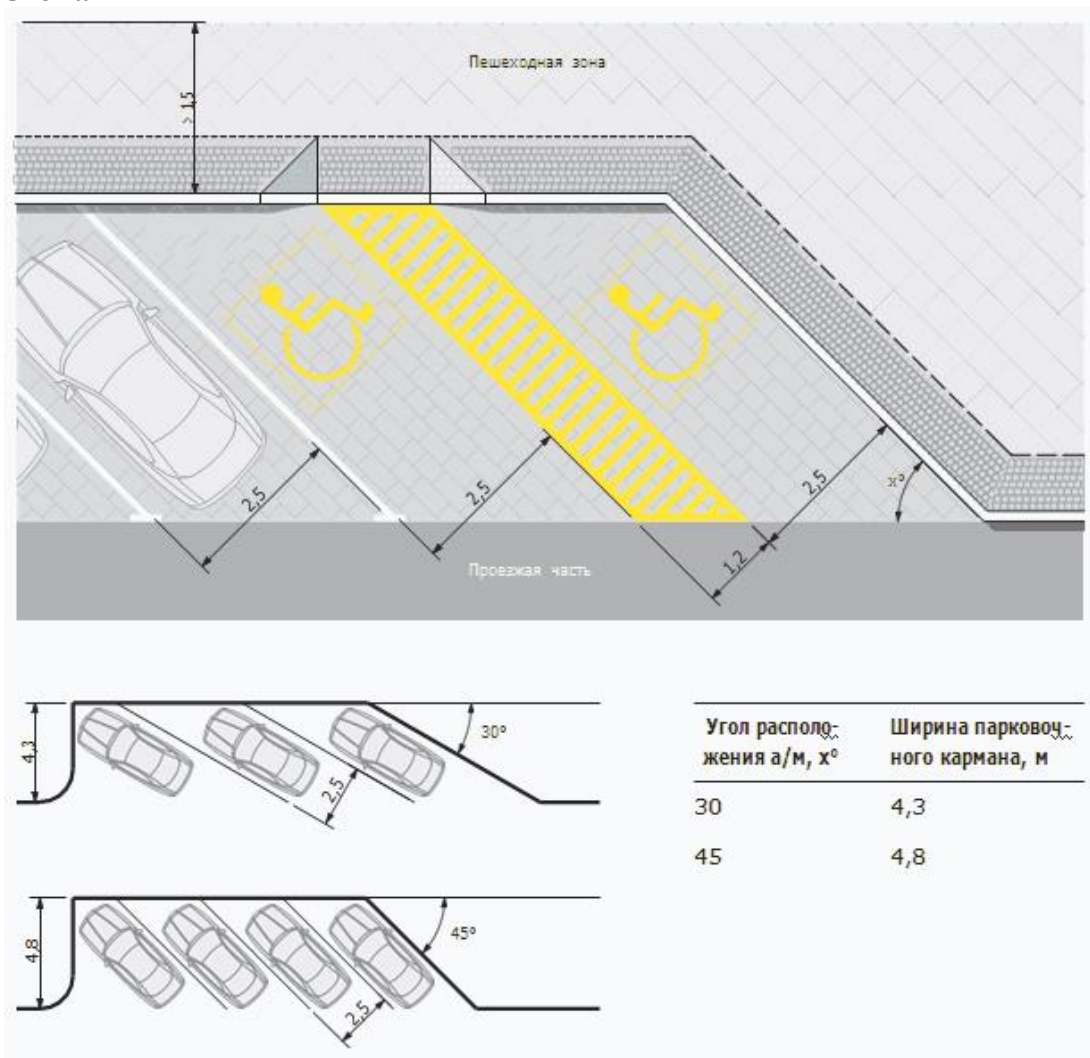
Схема 1
