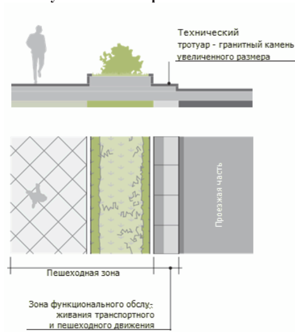
Технический тротуар, примыкающий к газону с высоким бортом
