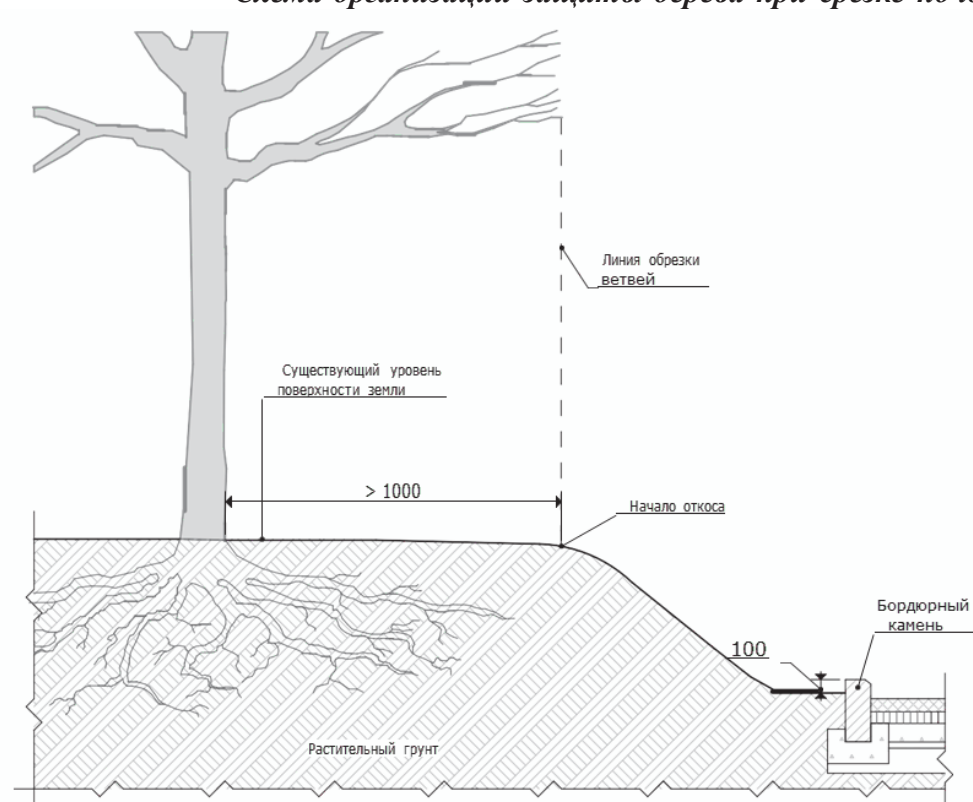
Схема организации защиты дерева при срезке почвы
