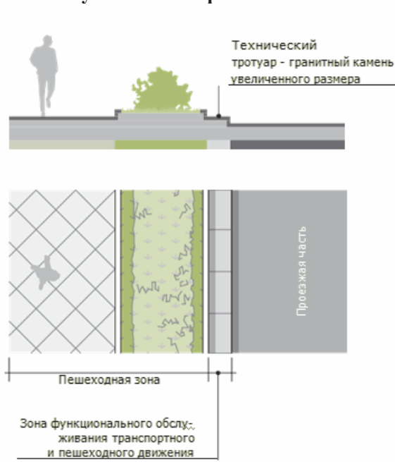
Технический тротуар, примыкающий к газону с низким бортом
