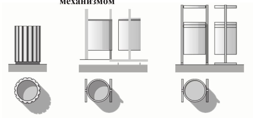
Примеры размещения урн
