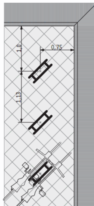
Велопарковка, расположенная под углом 45°
