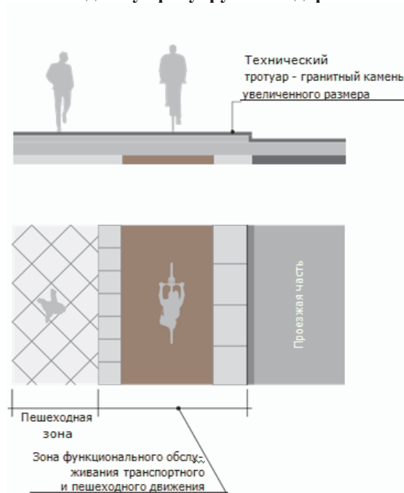
Технический тротуар, примыкающий к пешеходному тротуару и велодорожке
