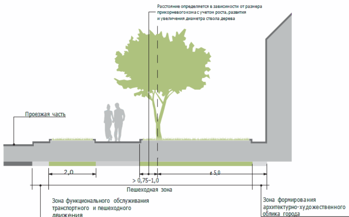
Схема 4
