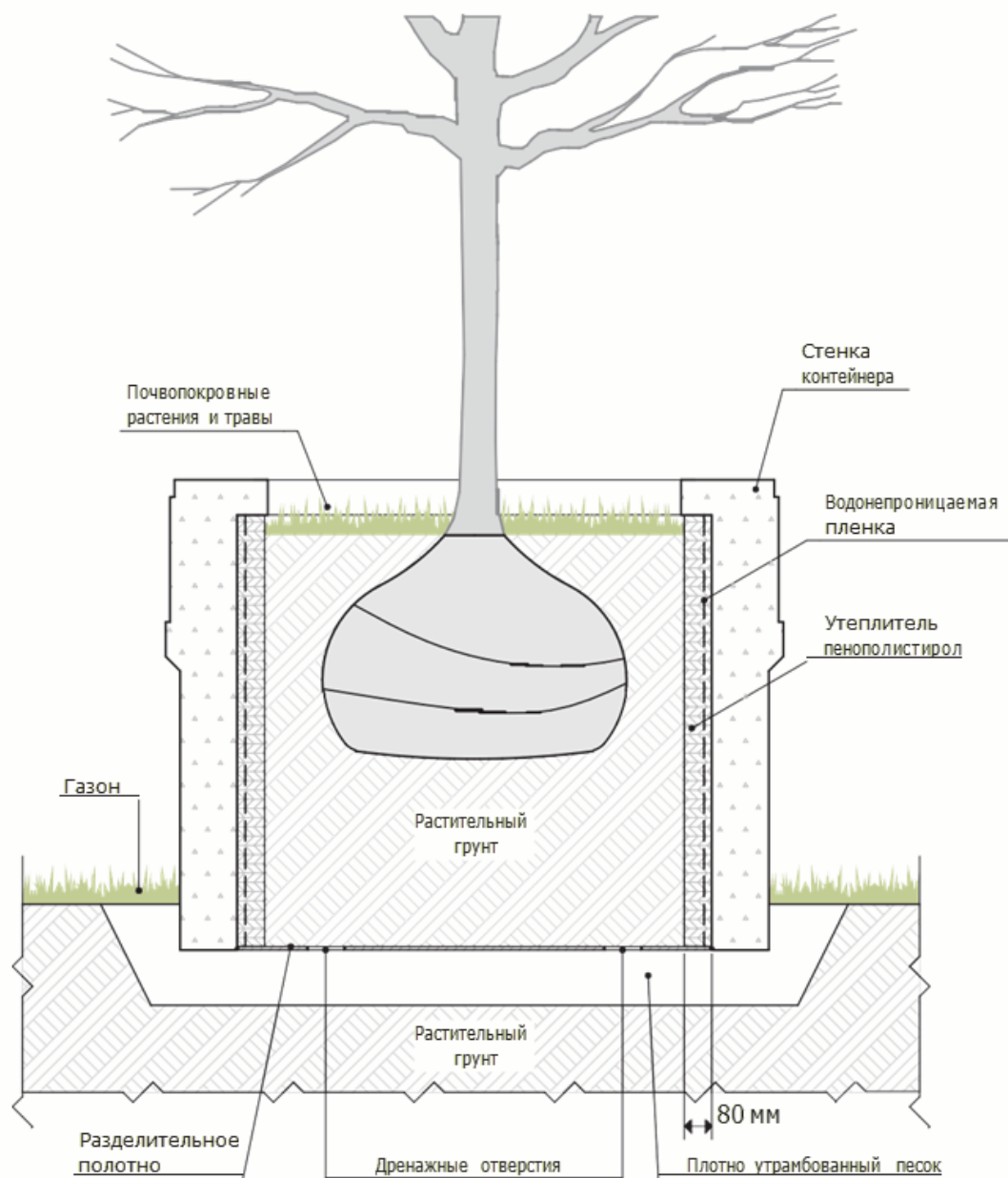
Схема организации посадочного места с наземным размещением контейнера
