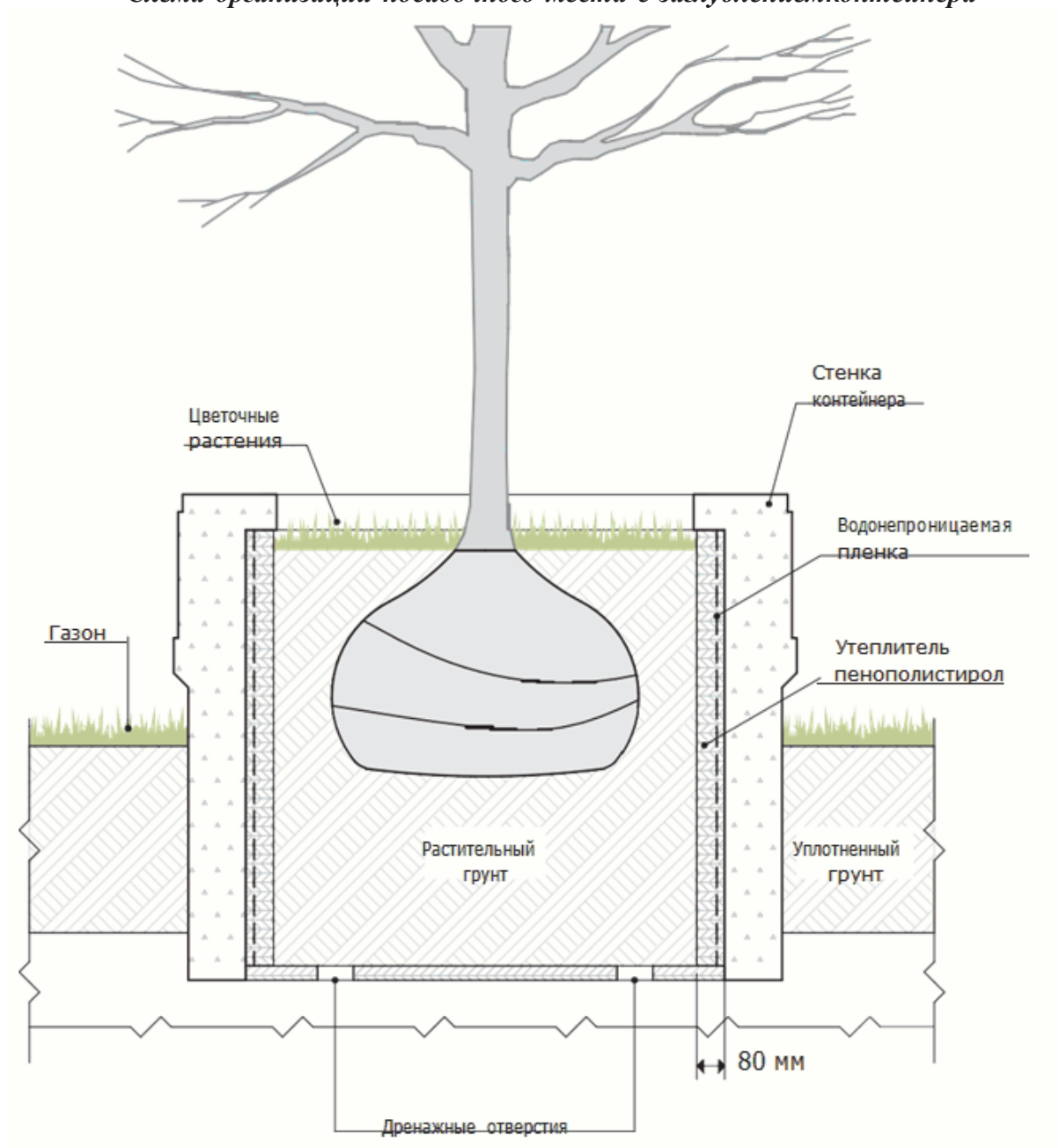
Схема организации посадочного места с заглублением контейнера
