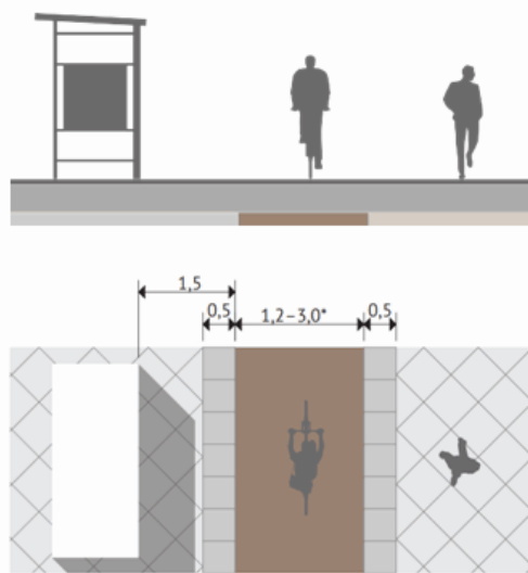
Размещение велодорожки между остановкой и пешеходной частью
