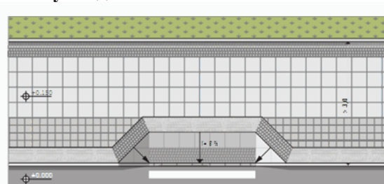
Схема 3–2. Пример организации предупреждающих покрытий при помощи изменения цвета, фактуры и типа укладки
