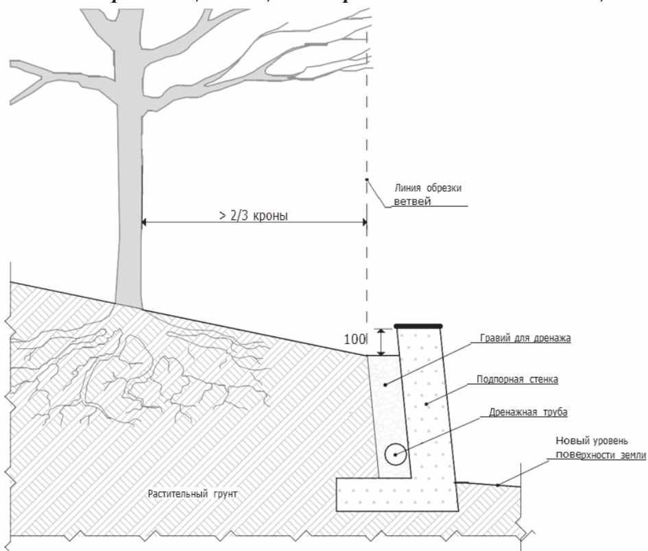
Схема организации защиты деревьев на склоне с помощью подпорной стенки
