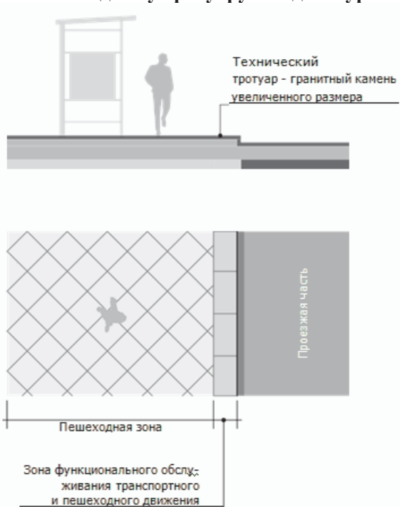
Технический тротуар, примыкающий к пешеходному тротуару на одном уровне
